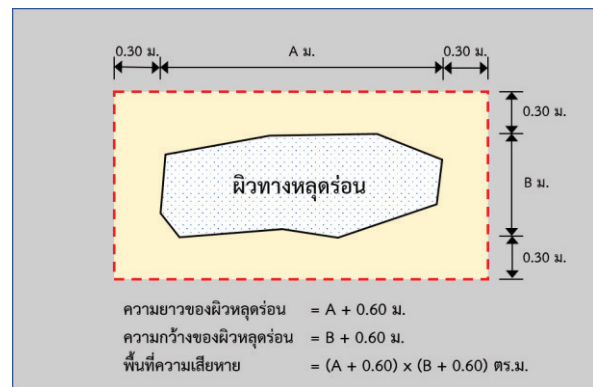
รูปที่ 4.4 ลักษณะความเสียหายแบบผิวทางหลุดร่อนและรูปแบบการวัดพื้นที่ความเสียหาย
